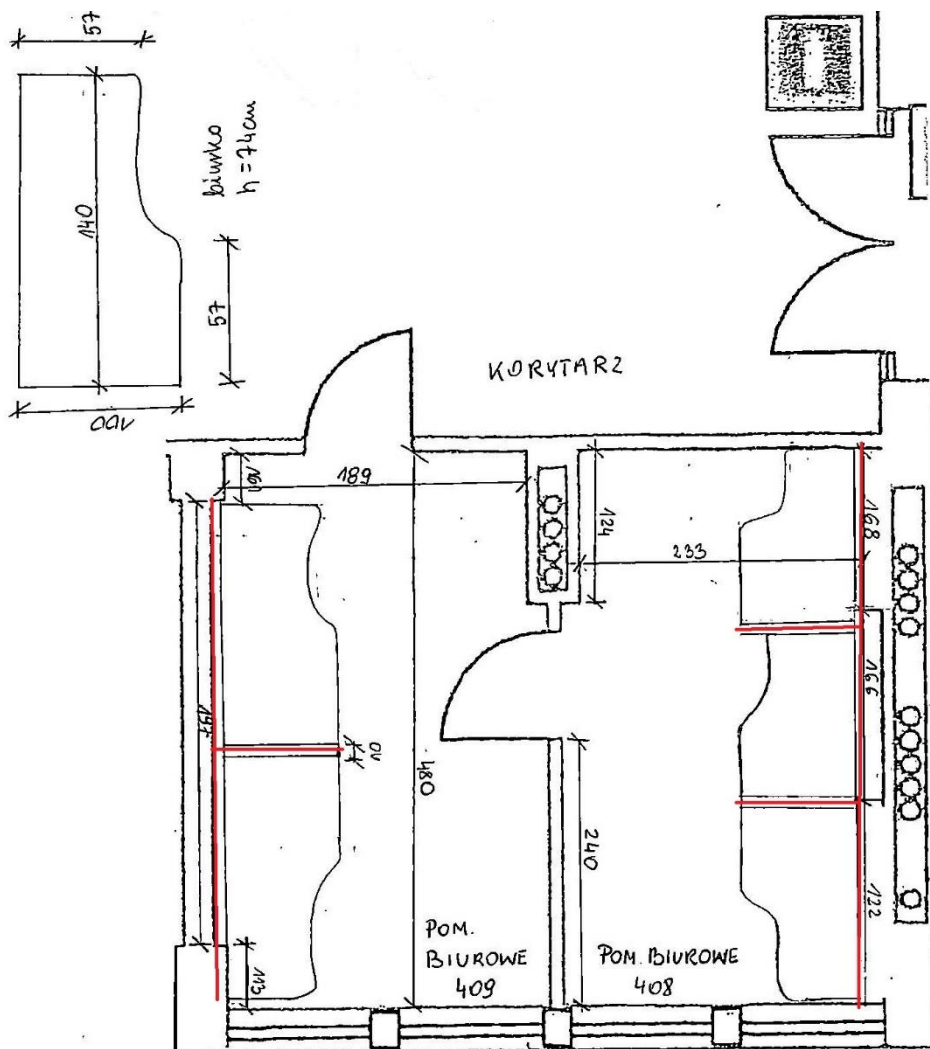
Rozmieszczenie ścianek działowych w Delegaturze Krajowej Informacji Skarbowej w Płocku
